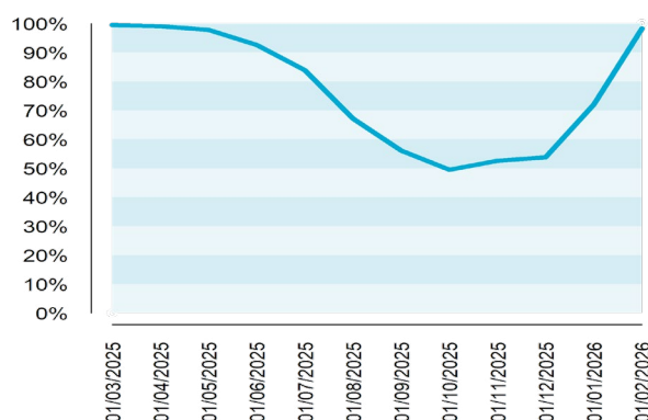
Retenue d'eau de Michelbach (7.3 M de m³)
