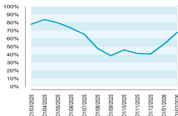
Retenue d'eau de Kruth-Wildenstein (11.6 M de m³)
