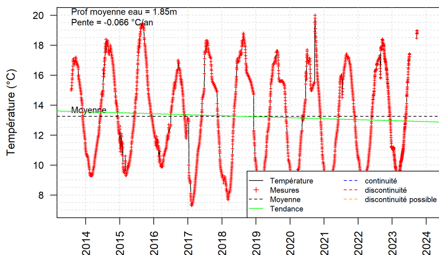
Figure 14 : Evolution de la température à Altorf (02714X0219/PZ)
