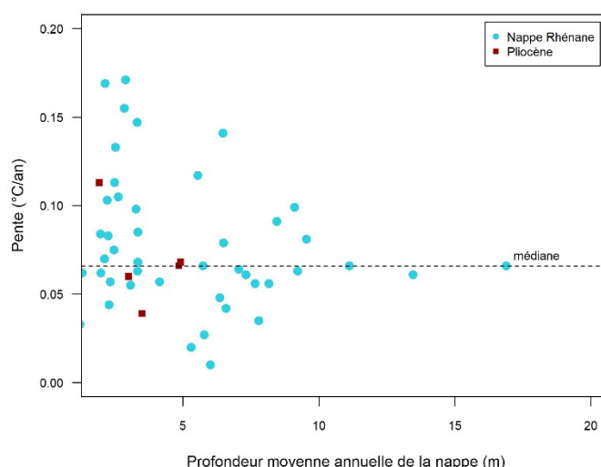
Figure 12 : Pente (°C/an) en fonction de la profondeur moyenne annuelle de la nappe (m)
