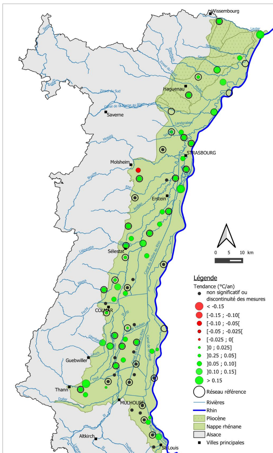
Carte 6: Evolution de la température (durée du suivi \geq 5 ans)
