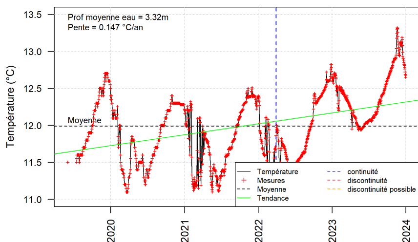
Figure 15 : Evolution de la température à Offendorf (02351X0340/320A)
