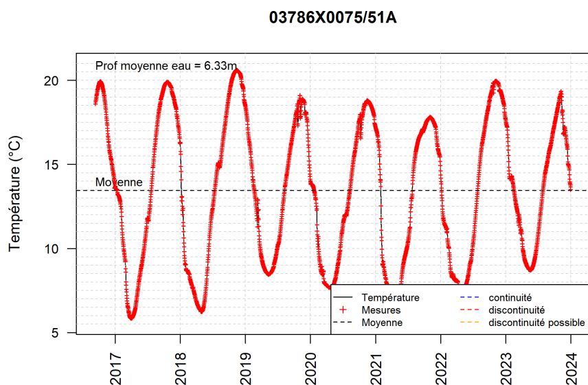
Figure 19 : Evolution de la température à Réguisheim (03786X0075/51A)
