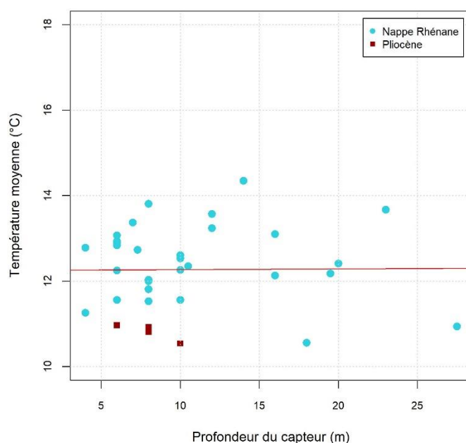
Figure 8 : Températures moyennes annuelles en fonction de la profondeur du capteur
