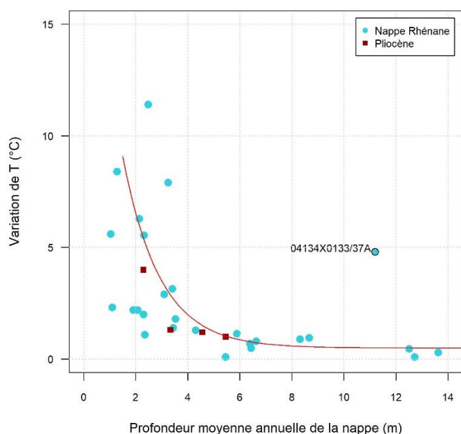
Figure 7 : Amplitude des variations annuelles de température en fonction de la profondeur moyenne de nappe par rapport au sol
